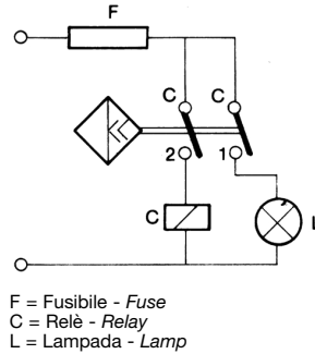
Schema di applicazione Application chart
