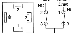
Collegamenti elettrici standard Standard electrical connection
