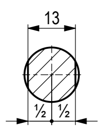
ŘEZ A-A
